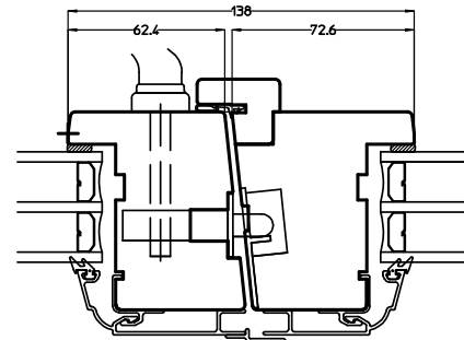
Horizontalsnitt mötesbåge
