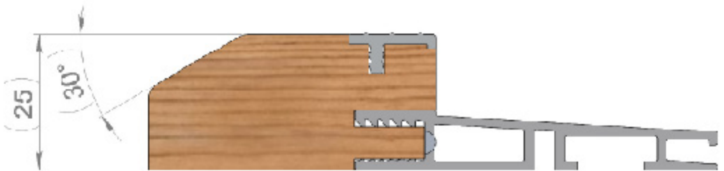
Standardtröskel, ek/alu
